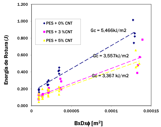
Figura 12. Cálculo del valor G_c mediante el método de Plati y Williams, para los compuestos de PES/MWCNT.
