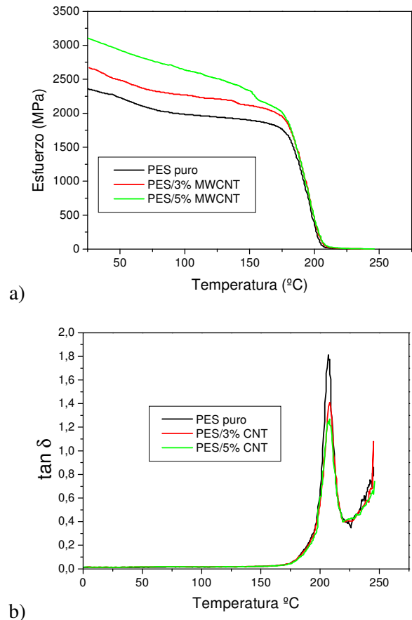
Figura 6. Representación gráfica de las propiedades visco-elásticas en el DMA para el PES y sus compuestos PES/CNT a) Módulo de almacenamiento b) \tan \delta
