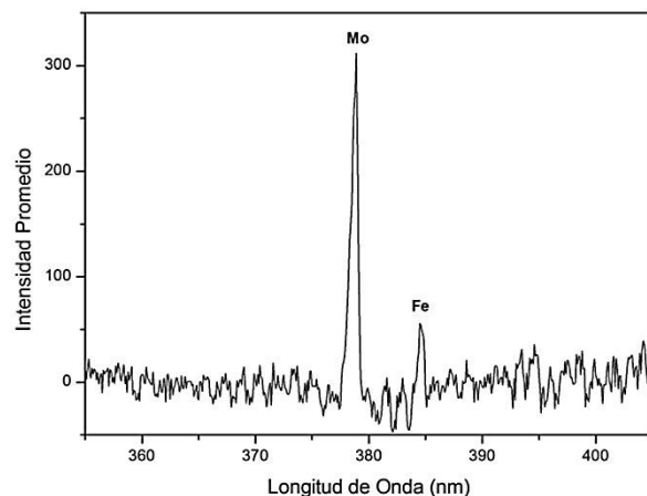
Figura 5. Espectros de emisión para el Naranja de Molibdeno (Resina/Vidrio) (1 pulso)
