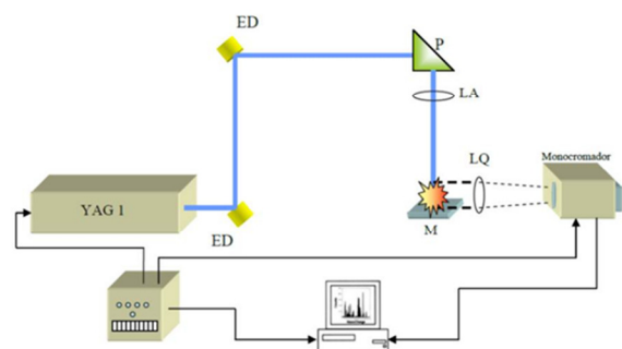
Figura 1. Montaje experimental.
