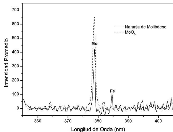
Figura 2. Espectros de emisión comparados para el Naranja de Molibdeno y el patrón de \text{MoO}_3 (10 pulsos).
