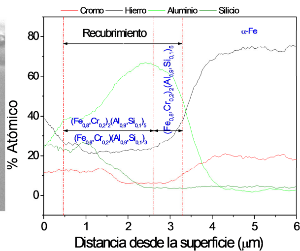
Figura 3. Micrografías y análisis lineal del corte transversal del recubrimiento de Al-Si sobre el acero HCM-12A durante 90 minutos a) 520 °C, b) 550 °C y c) 580 °C.
