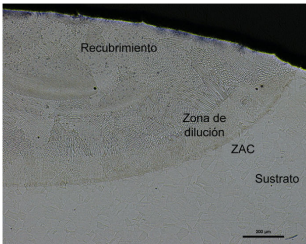
Figura 3. Micrografía óptica de recubrimiento procesado a 300 mm/min, 40 mg/s y 1.2 kW (Glyceregia, 50X), donde se aprecia el recubrimiento, la zona de dilución, la zona afectada por el calor y el sustrato.
