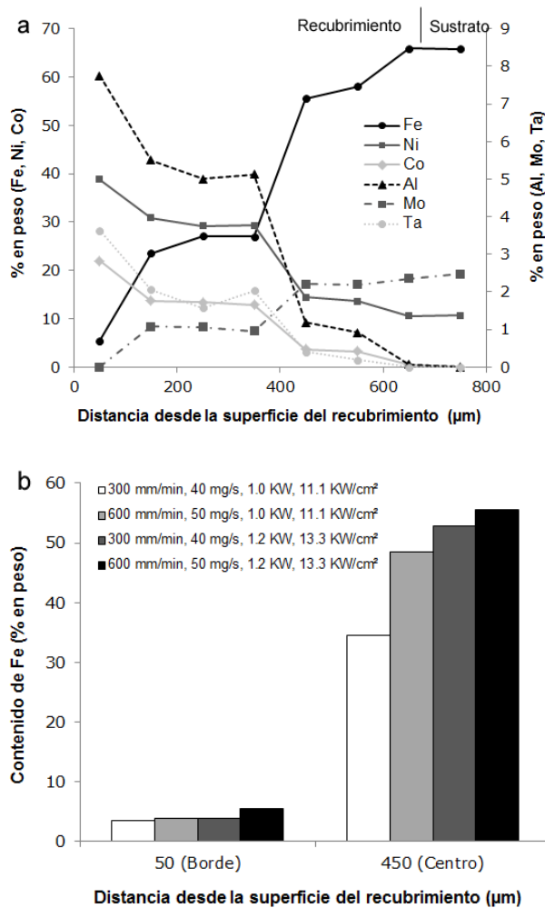
Figura 6. Evolución de la composición química, a) Recubrimiento procesado a 600 mm/min, 50 mg/s y 1,2 kW y b) Contenido de Fe en borde y centro del recubrimiento para cuatro condiciones.
