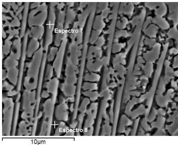
Figura 8. Detalle de dendritas columnares y celulares encontradas a 450 \mu\text{m} de la superficie del recubrimiento procesado a 600 mm/min, 50 mg/s y 1,0 kW.
