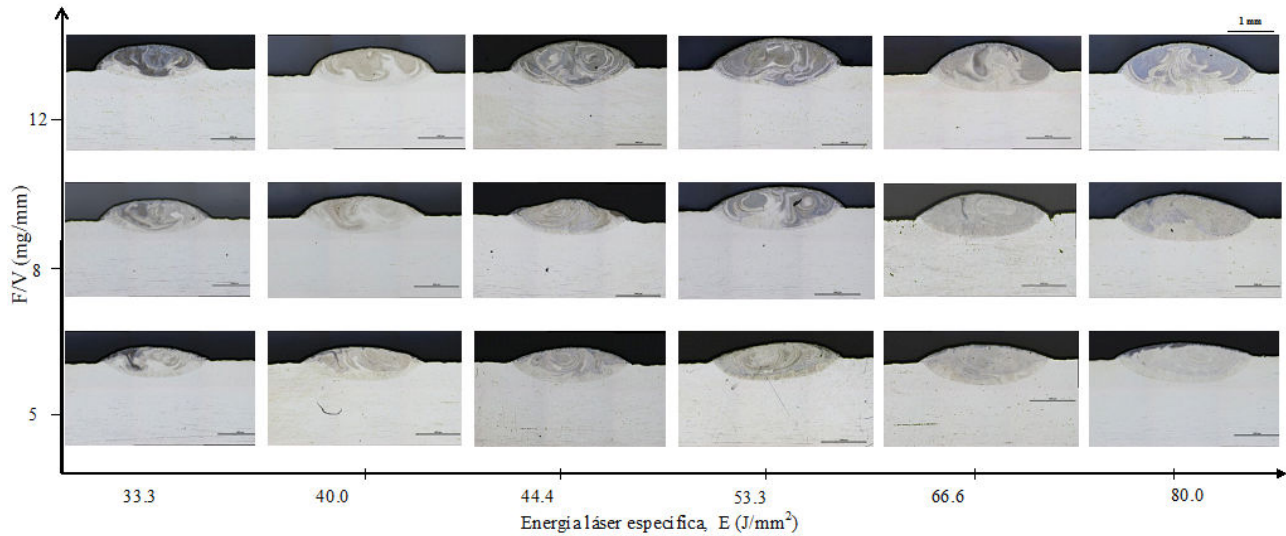
Figura 2. Mapa de proceso con las micrografías de los recubrimientos obtenidos por láser en función de la cantidad de polvo aportado por unidad de longitud y la energía láser especificada.
