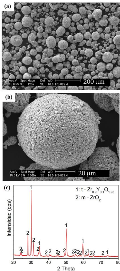
Figura 2. Morfología del polvo de circonita-itria-HCS: (a) Partículas vista general, 125X (b) Magnificación de una partícula, 1000X. (c) Espectro de DRX del polvo.
