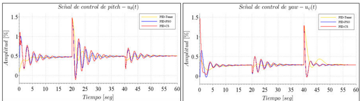
Figura 4. Señales de control u_{\theta}(t) (arriba) y u_{\psi}(t) (abajo) obtenidas con los controladores sintonizados con PID Tuner , PSO y CS .
