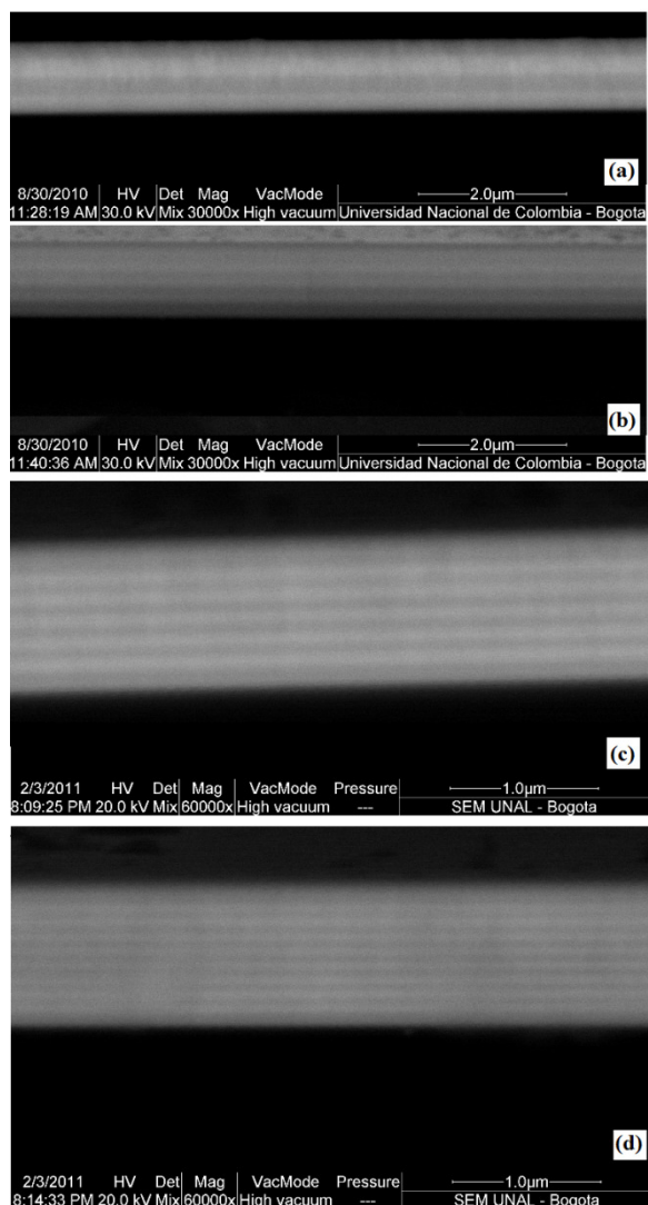
Figura 4. Sección transversal de las multicapas de (a) 2 bicapas, (b) 5 bicapas, (c) 7 bicapas y (d) 10 bicapas.
