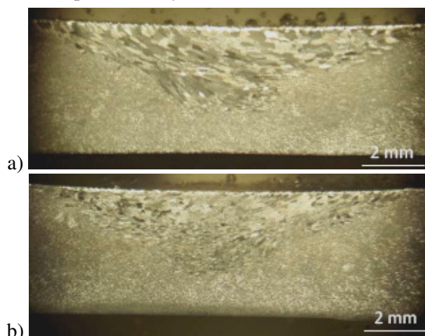
Figura 12. Muestras procesadas de AA7075 a 500°C: a- A2 (514/51), b- B2 (388/51).
