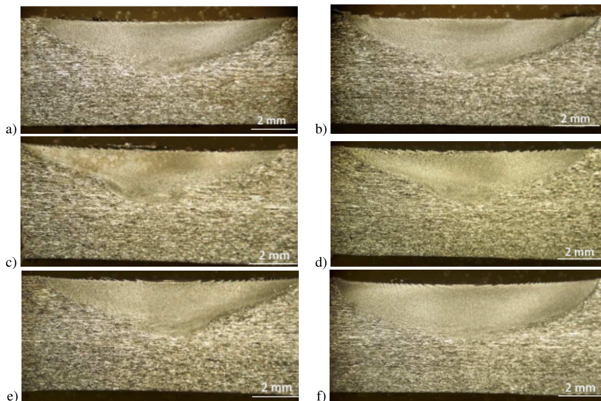
Figura 5. Muestras procesadas de AA5088 recocidas a 350°C: a- A1 (514/35), b- A2 (514/51), c- A4 (514/98), d- B2 (388/51), e- B3 (388/73), f- B4 (388/98).
