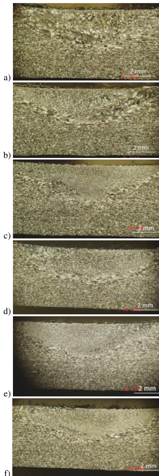
Figura 11. Muestras procesadas de AA5088 a 500°C: a- A1 (514/35), b- A2 (514/51), c- A4 (514/98), d- B2 (388/51), e- B3 (388/73), f- B4 (388/98).
