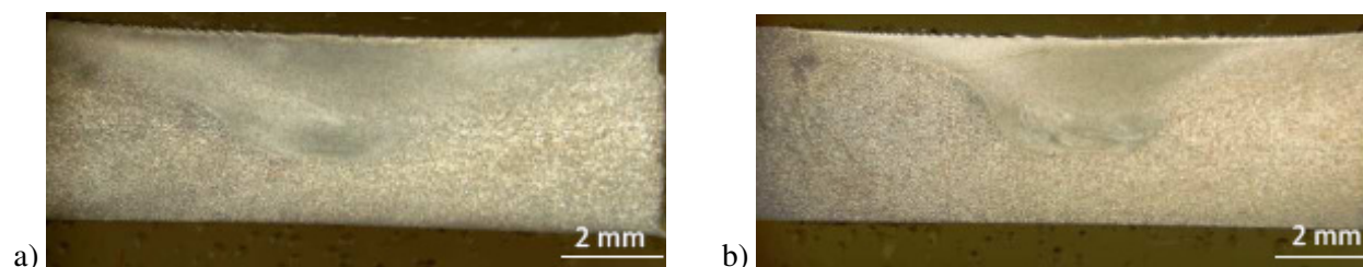
Figura 6. Muestras procesadas de AA7075 a 350°C: a- A2 (514/51), b- B2 (388/51).
