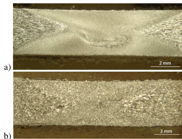
Figura 4. Macrográficas de 5088-A3 y recocida: a- 350°C y b-550°C.
