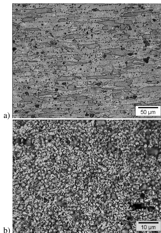
Figura 2. Micrografías: a- material base 7075 y b- material procesado 7075- B2 (388/51).
