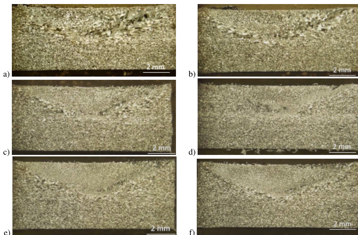
Figura 9. Muestras procesadas de AA5088 a 450°C: a- A1 (514/35), b- A2 (514/51), c- A4 (514/98), d- B2 (388/51), e- B3 (388/73), f- B4 (388/98).
