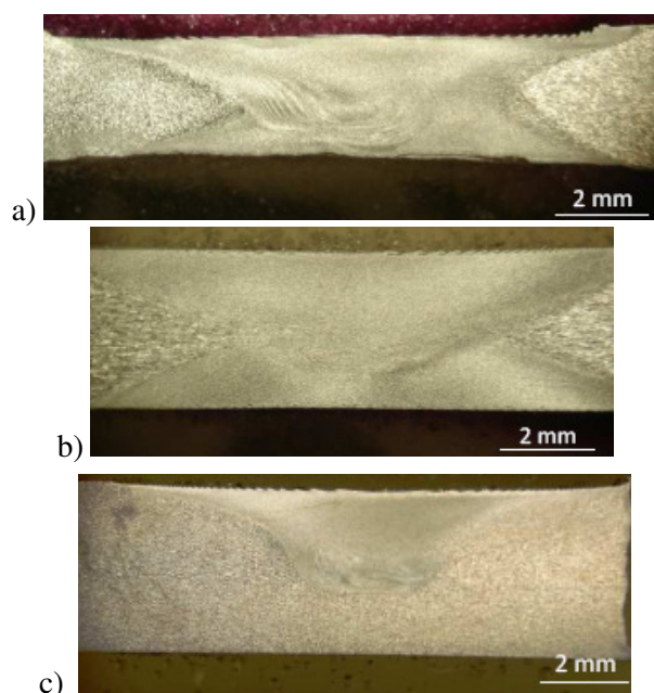
Figura 1. Macrografías de probetas procesadas por FSP: a- 5052 (2 pas.), b-5088 (2 pas.) y c-7075 (1 pas.).
