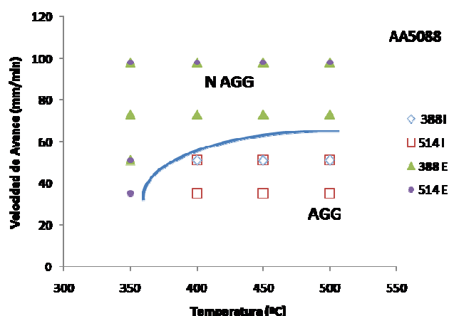
Figura 13. Efecto de los parámetros de procesamiento FSP sobre la estabilidad térmica de AA5088, en función de la temperatura de recocido.
