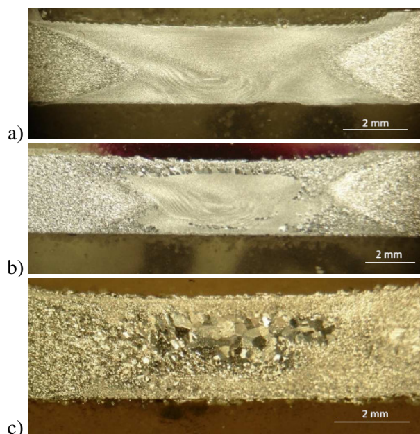
Figura 3. Macrográficas de 5052-A5 recocida: a- 310°C, b- 350°C y c-400°C.
