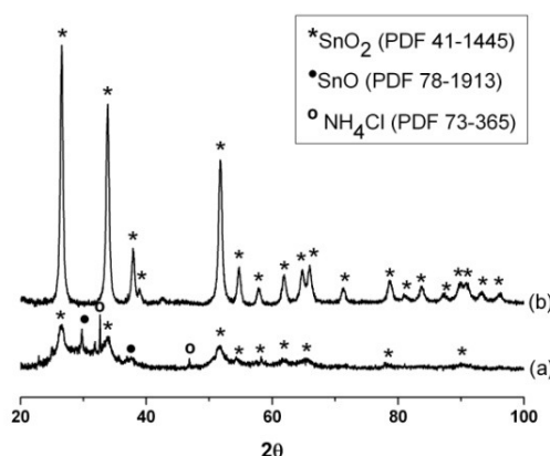
Figura 6. Difractograma de rayos X correspondiente a una muestra sólida del sistema \text{SnCl}_2\text{-H}_2\text{O-NH}_4\text{OH} : (a) obtenido a pH 4.2, sin envejecer, y (b) lavada con una solución de dietilamina 0.5M, tratada térmicamente a 500^\circ\text{C} .
