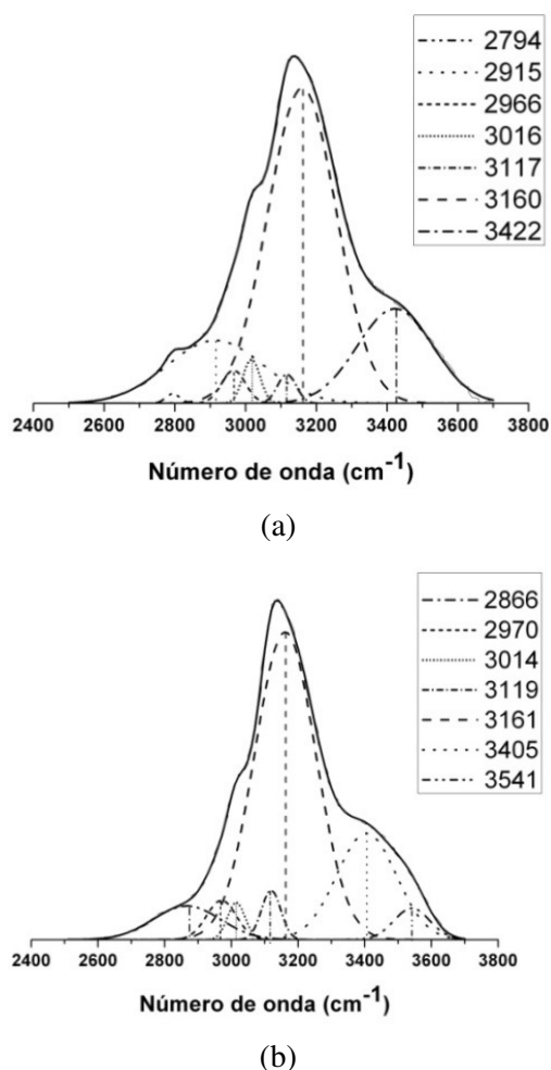
Figura 5. Deconvolución de la banda espectral de la zona 2 (entre 3000 y 3650\text{ cm}^{-1} ) correspondiente a muestras sólidas del sistema \text{SnCl}_2\text{-H}_2\text{O-NH}_4\text{OH} : (a) sin envejecer y (b) envejecido 15 días (pH de 4.2).
