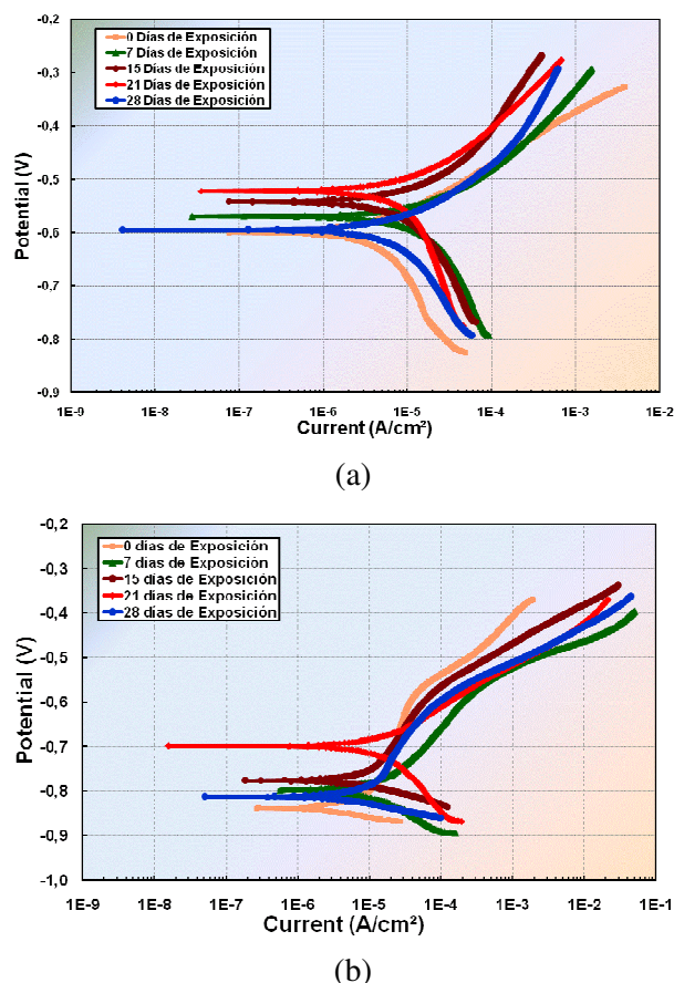
Figura 2. Curvas de extrapolación de Tafel en muestras (a) implantadas con iones de Ti a 5 keV y (b) sin tratamiento superficial, inmersos en solución de NaCl al 3 %wt., de 0 a 672 horas.
