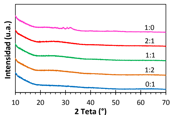
Figura 1. Difractogramas de rayos x de los polvos de biovidrio/Al 2 O 3 calcinados a 700°C.
