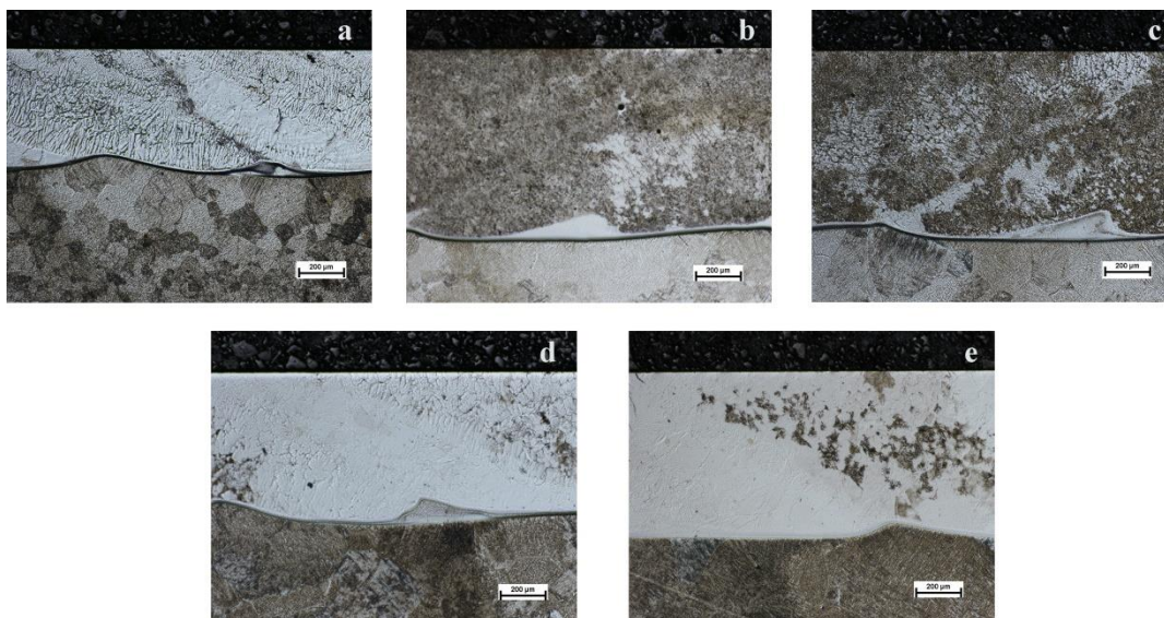
Figura 2. Micrografías obtenidas por microscopía óptica de los recubrimientos efectuados rectificadas: a) R01, b) R02, c) R03, d) R04 y e) R05.
