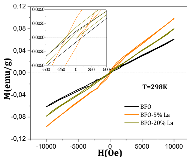
Figura 9. Curvas M-H obtenidas para el sistema \text{Bi}_{1-x}\text{La}_x\text{FeO}_3 con x=0.0 , 0.15 y 0.20 tratadas térmicamente a 750^\circ\text{C} durante 3 horas.
